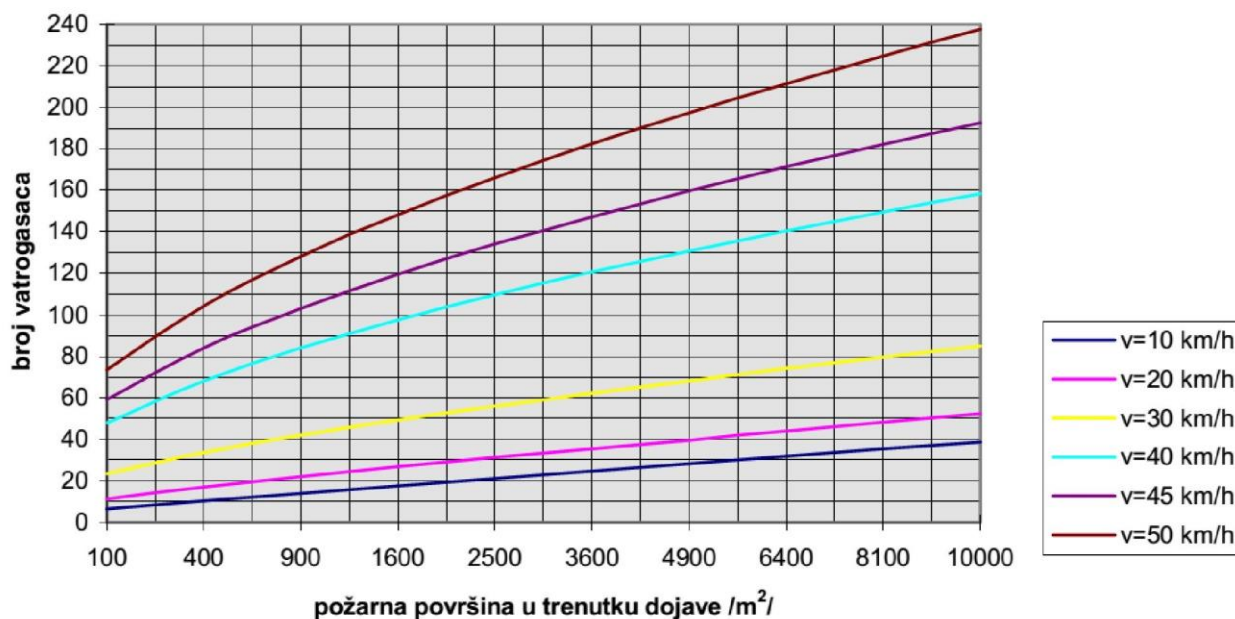
Slika 4: Grafički prikaz potrebnog broja vatrogasaca N_v za gašenje požara otvorenih prostora u periodu intervencije t=15 min, pri brzini vjetra v=10-50 km/h
