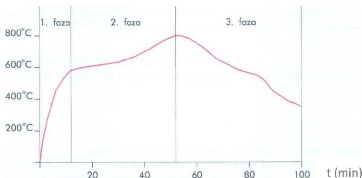
Slika 2: Razvoj tipičnog požara
